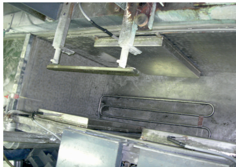
VASCA CON TRASDUTTORI IMMERGIBILI IN IMPIANTO GALVANICO
